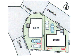
配置図
