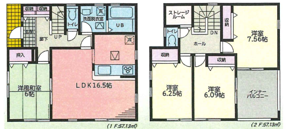
1号棟間取図
